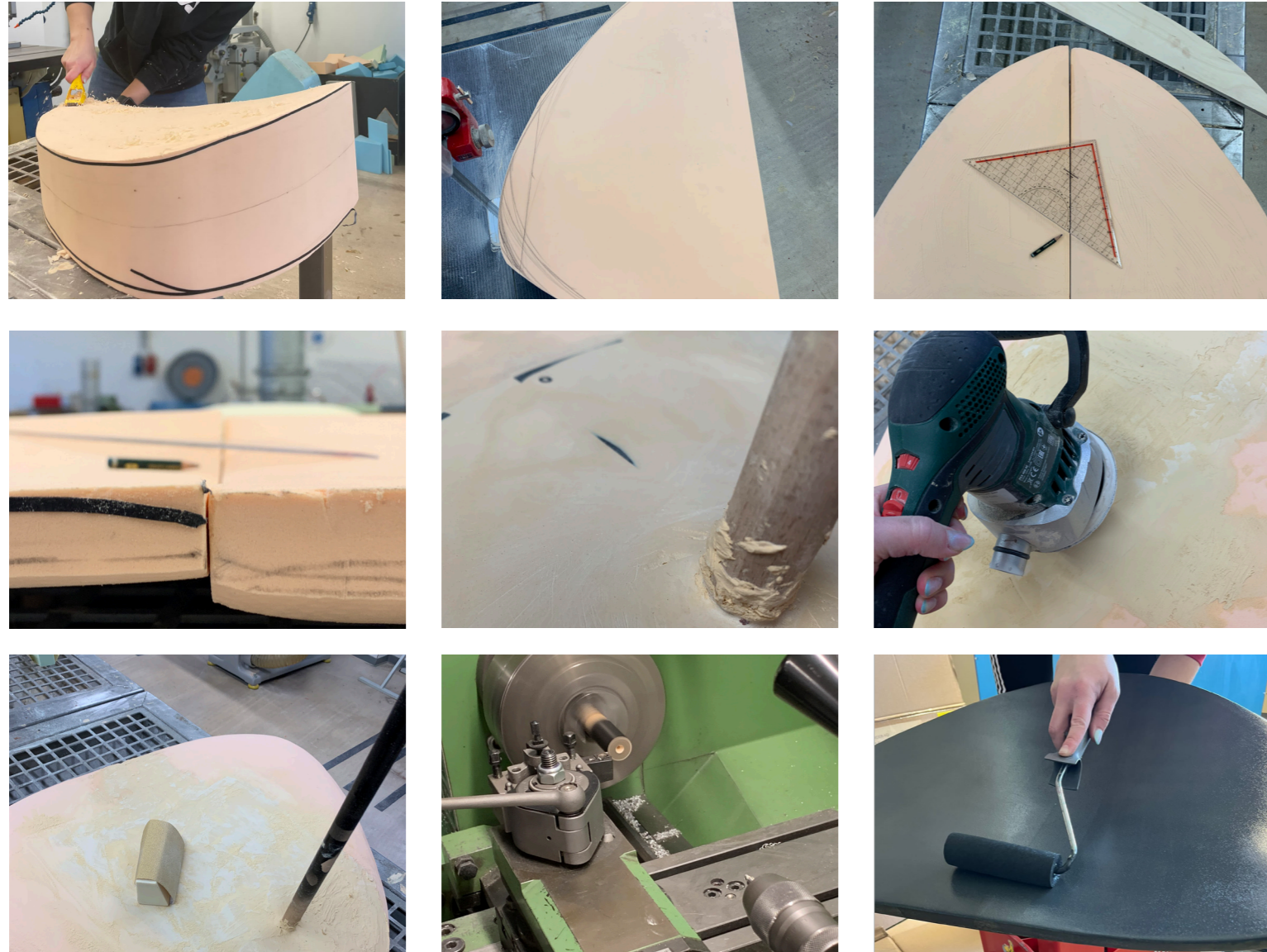
Dach aus Polystyrol formen, schleifen und lackieren
